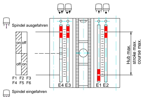
Bild / figure 1 : Einstellung der Wegschalter und Endlagenschalter / Adjustment of limit switches and switches for intermediate position / Réglage des positions intermédiaires
