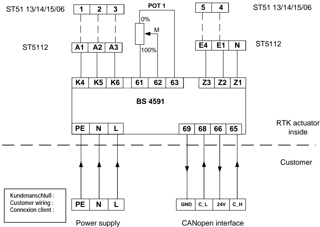
Anschlussplan ST 51xx / wiring diagram ST 51xx / schéma de câblage pour ST51xx
