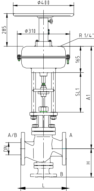
PV 6311/ PV 6321/ PV 6331, #150 / #300
