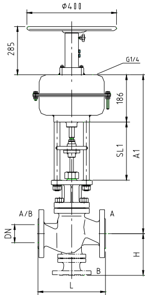
PV 6311/ PV 6321/ PV 6331, #150 / #300
