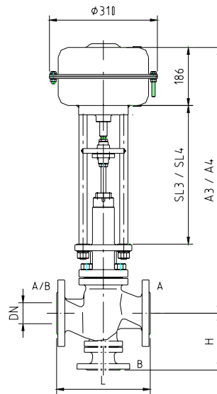
PV 6314/ PV 6324/ PV 6334, #150
