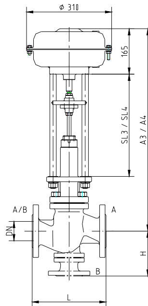
PV 6314/ PV 6324/ PV 6334, #150
