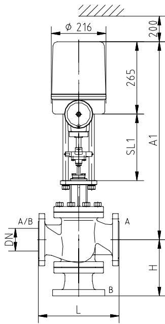
MV 5311/ MV 5321/ MV 5331, #150 / #300
