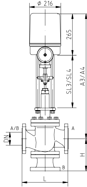
MV 5314/ MV 5324/ MV 5334, #150
